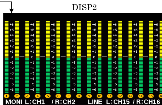
ピークメータ、VUメータの拡大表示
