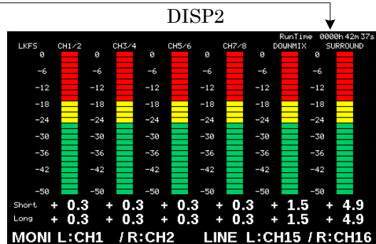
ラウドネスメータの表示
