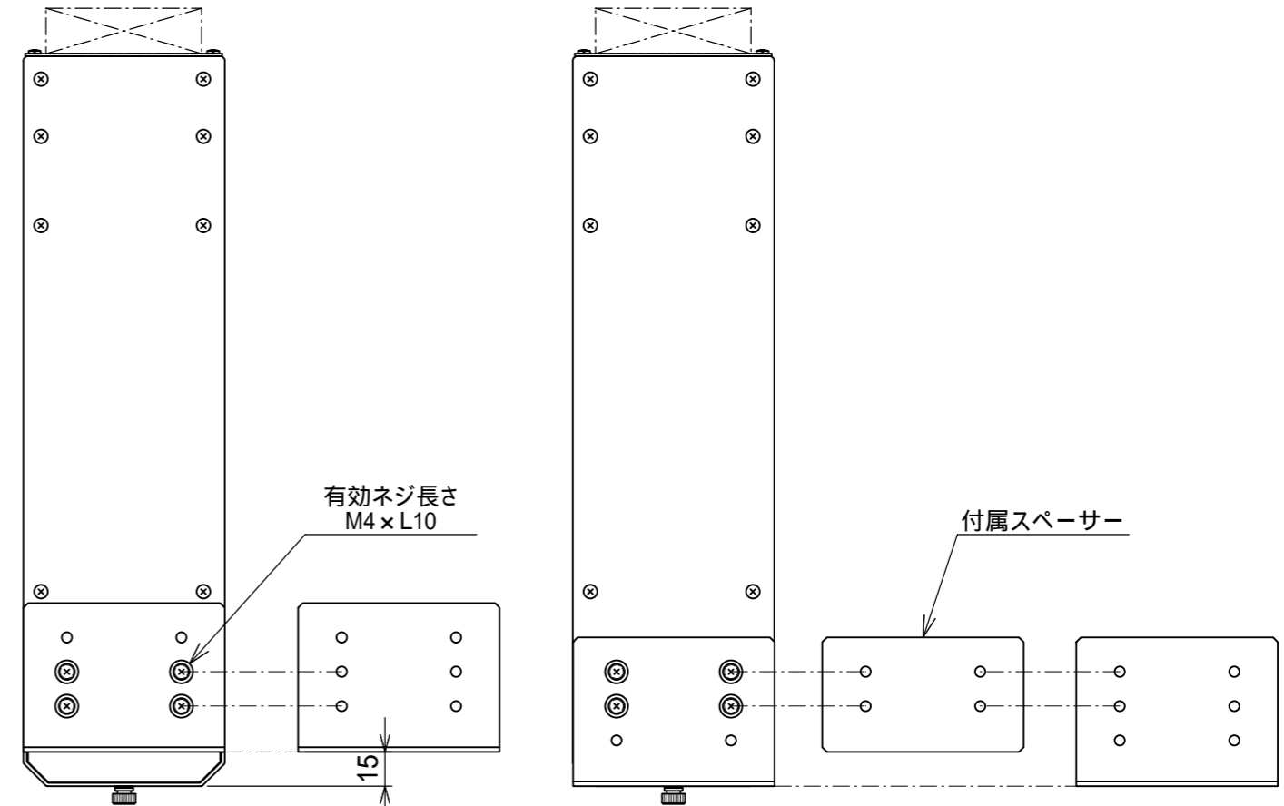
ラックマウント金具 [標準取付要領図]
