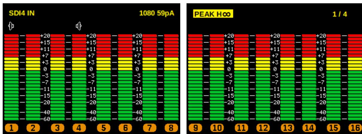
SDI4入力、ピークホールド \infty 表示、1/4chモニタリング,1~16ch表示
