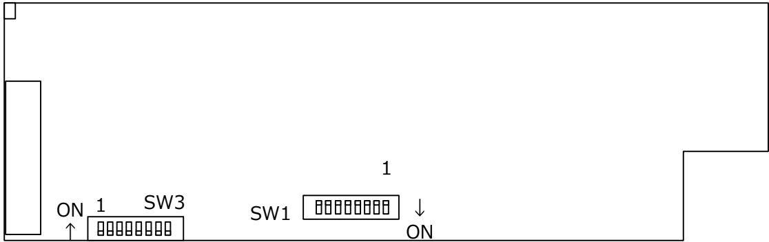
SW1
