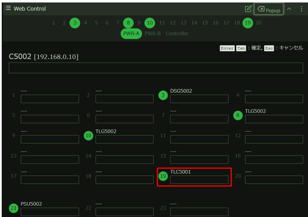
図 3-5 TLC5001 装着例
