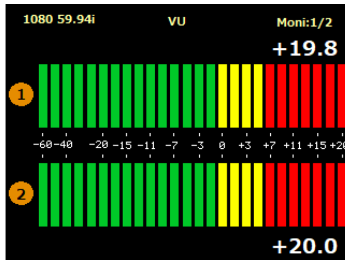
SDI入力、VU表示、レベル表示(L/R)
