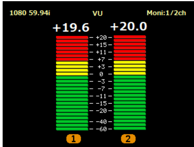
SDI入力、VU表示、2ch表示(L/R)
