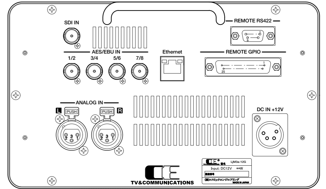
-背面図-
