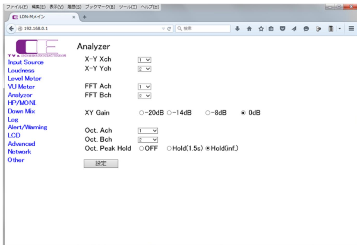
アナライザ設定画面
