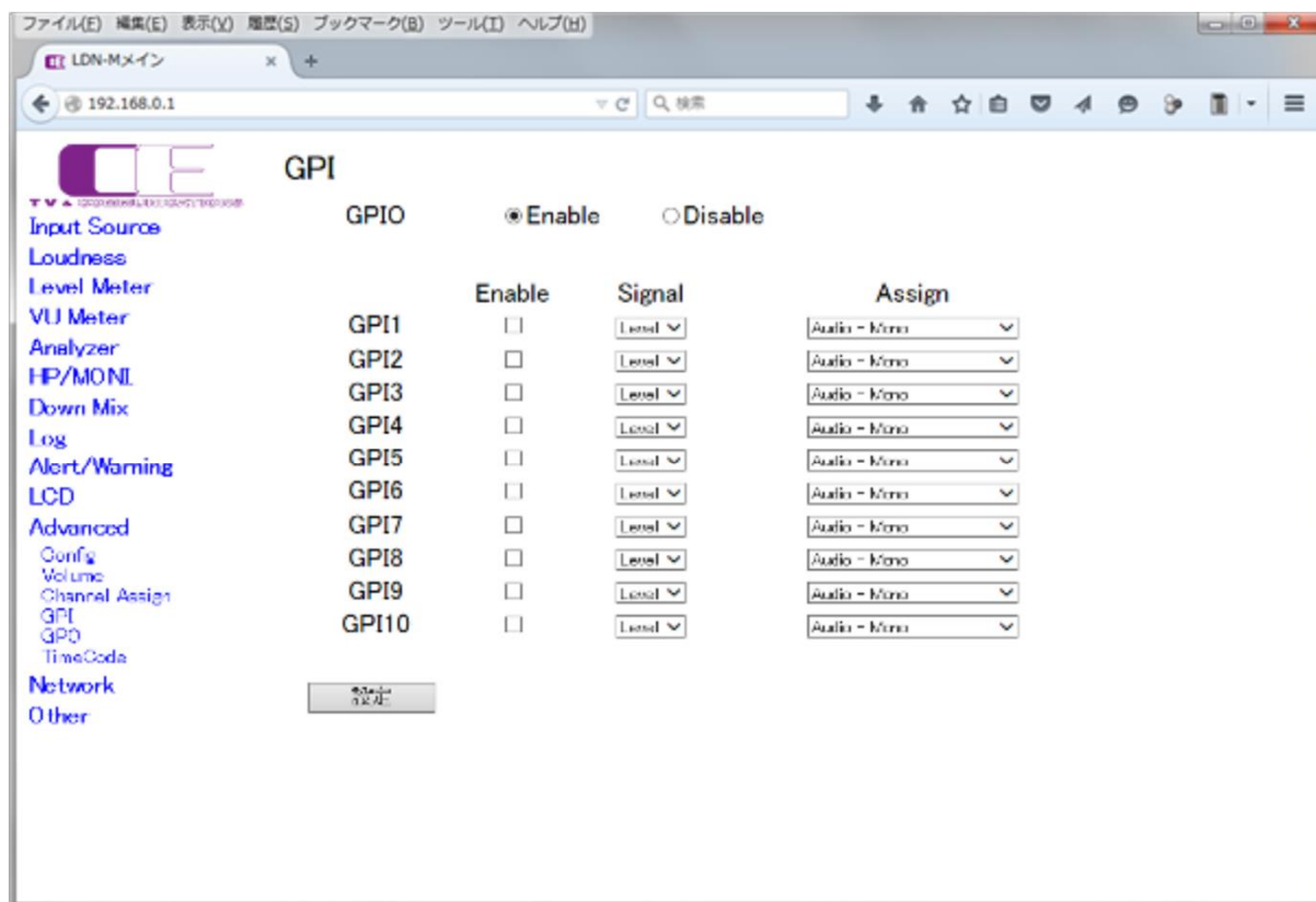
GPI設定画面
