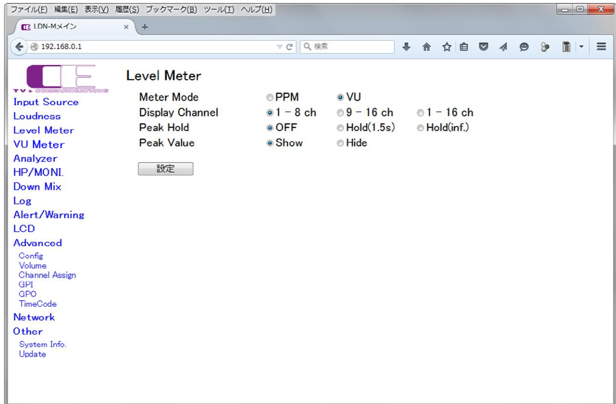
レベルメーター設定画面
