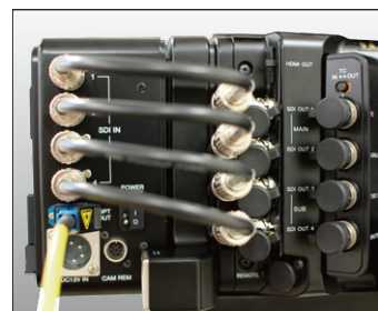
4K-EO 4K カメラとの接続例
