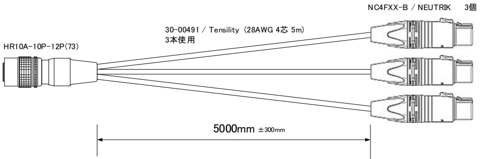
結線図
