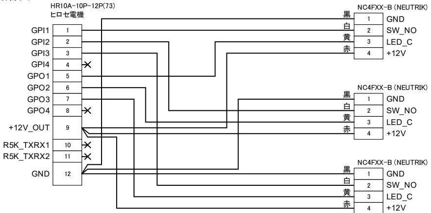
結線図
