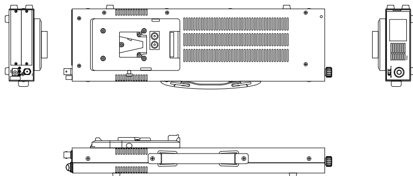
バッテリーアダプタを取付した状態
