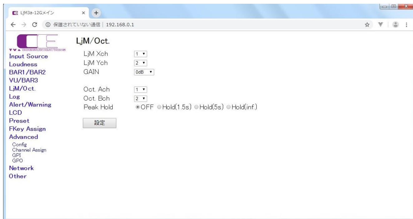
リサージュメーター／オクターブバンド設定画面
