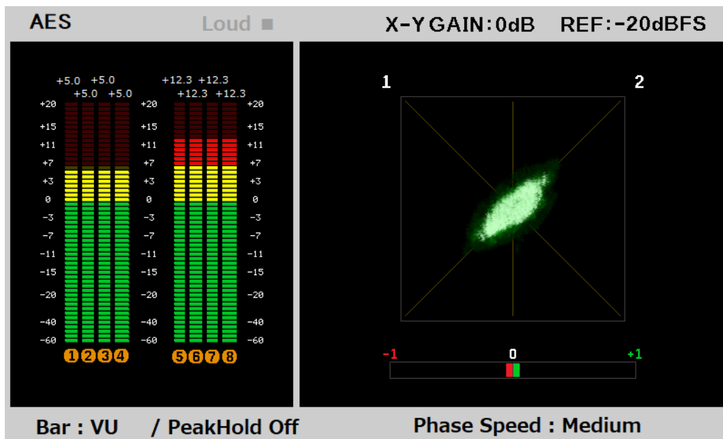
リサージュ、位相、バーグラフメーター表示
