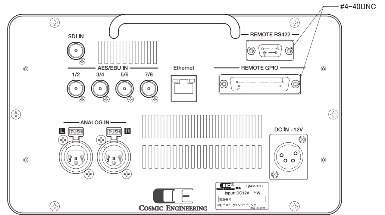
-背面図-
