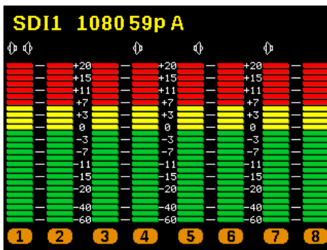
シングルソースモード、入力ソース SDI1, BAR 1-8, BAR 9-16 表示
