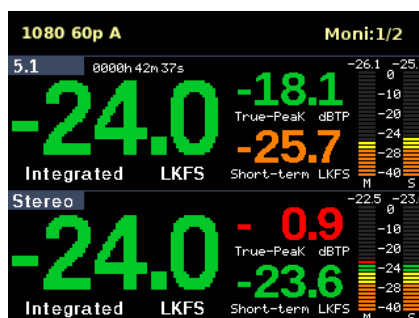
トゥルーピーク+ラウドネス
