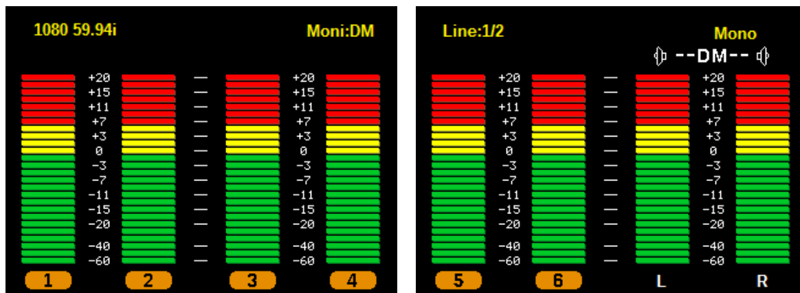
SDI1(SDI2) 1080i59.94 モニタチャンネル DM(ダウンミックス)、ライン出力チャンネル 1/2ch モノラルモード
