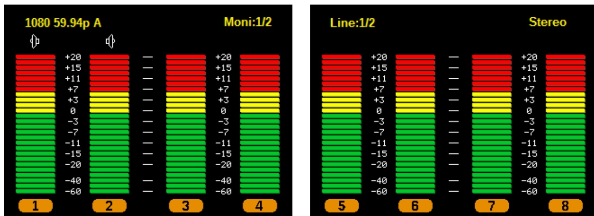
SDI1(SDI2) 1080p59.94 level A モニタチャンネル 1/2ch、ライン出力チャンネル 1/2ch ステレオモード
