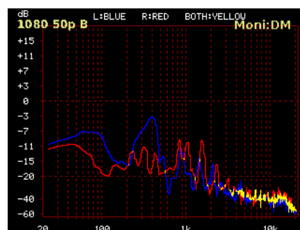
スペクトラムアナライザー
