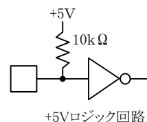
入力等価回路
