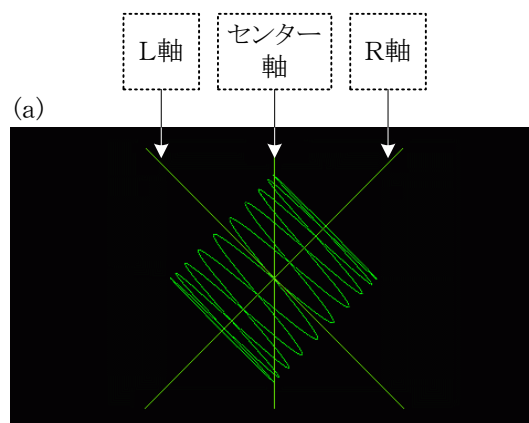
X-Yスコープの表示例
